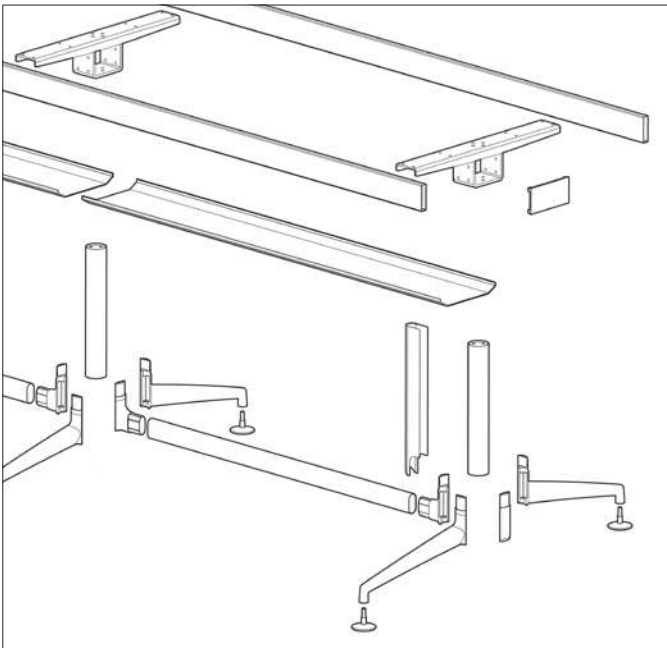
Das Prinzip von fina conference ist der modulare Aufbau des Gestells.
