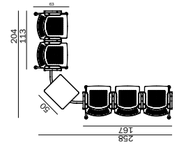
Konfigurationsbeispiel für Eckverbindung SE 00352/ Example of configuration of corner joint SE 00352
